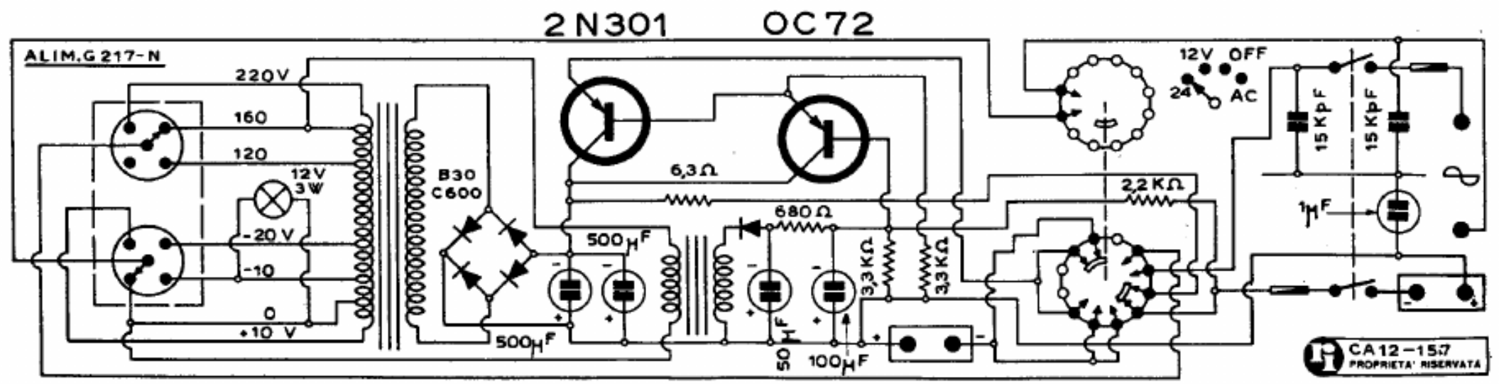
GELOSO S.p.A. - Amplificatore Mod. G 216 TSN
